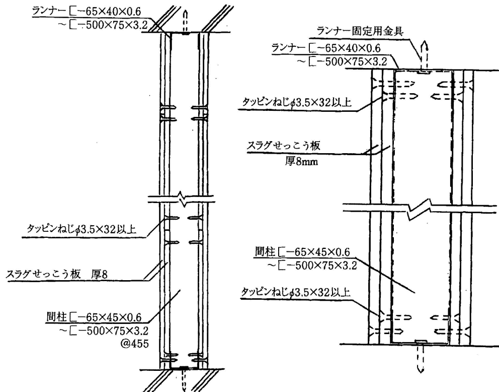
垂直断面図
