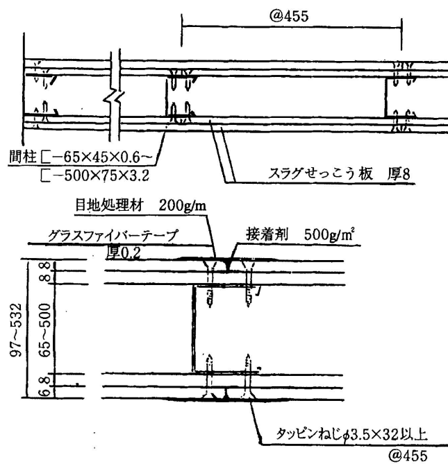
水平断面図
